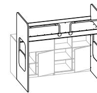
Рд 31.033 Кровать 1906х2072х973
