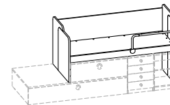
Рд 31.031П Рд 31.031Л Кровать 1274х2072х973
