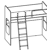
Рд 31.090П Рд 31.090Л Кровать 1906х2072х973
