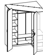
Рд 31.065П Рд 31.065Л Шкаф для одежды 2160х1637х1447
